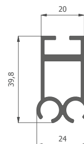
NF200 profil belki przeciwwietrznej
