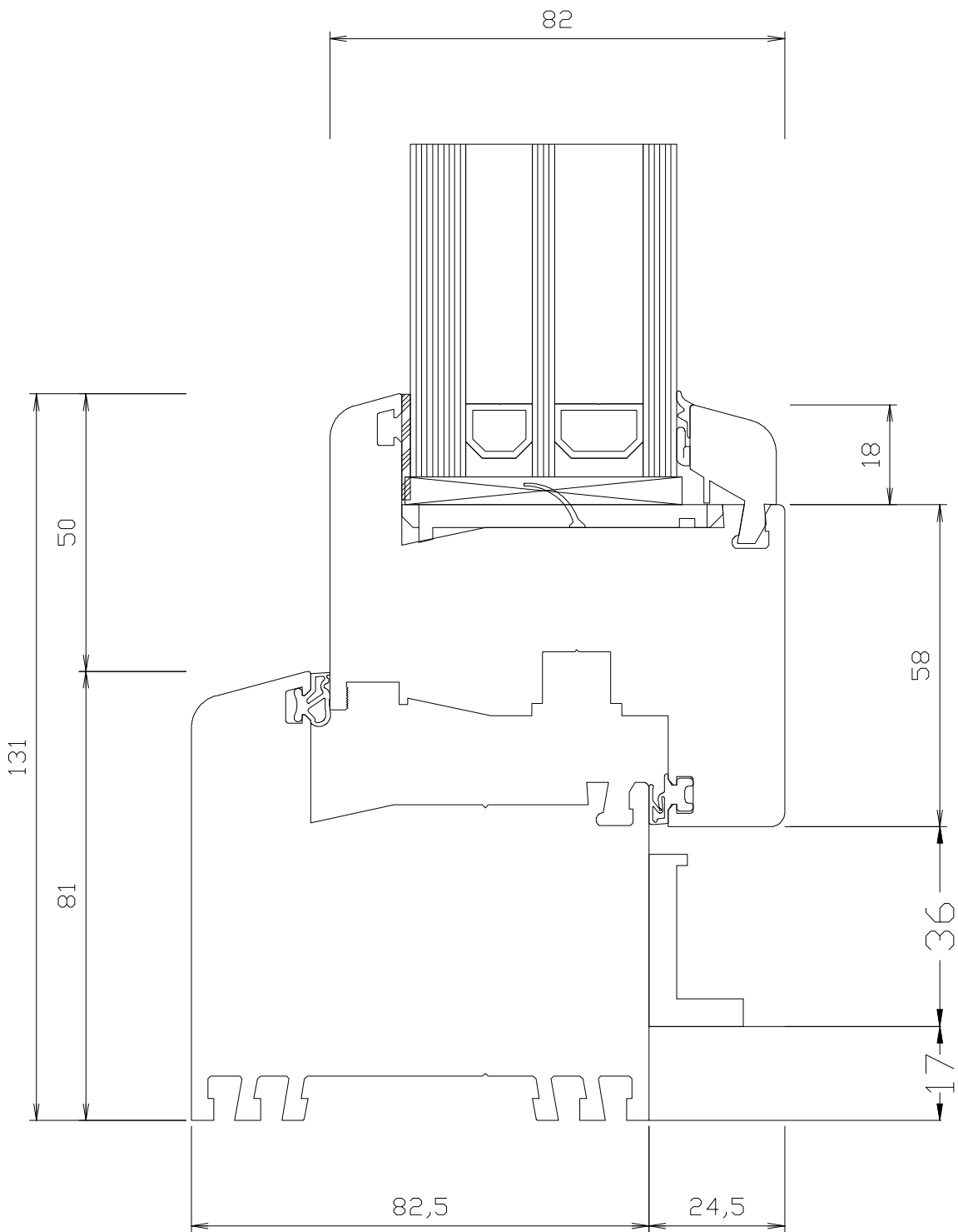
Szyna dolna okucia DuoPort
